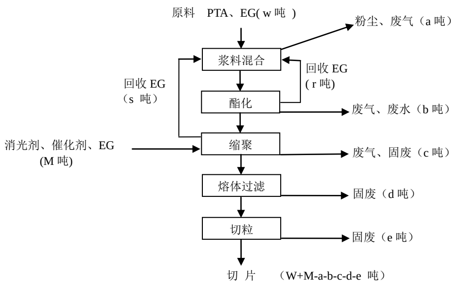
图 B.5 聚酯切片生产物料平衡示例图
