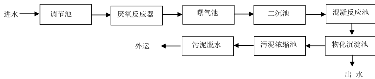
图 B.7 典型污水处理工艺流程示例图
